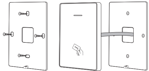
安装示意图
