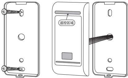
安装示意图
